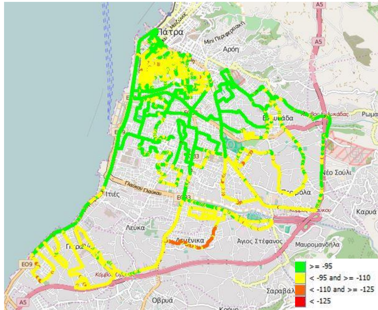
Εικόνα 13-3: Ραδιοκάλυψη Wind – LTE
