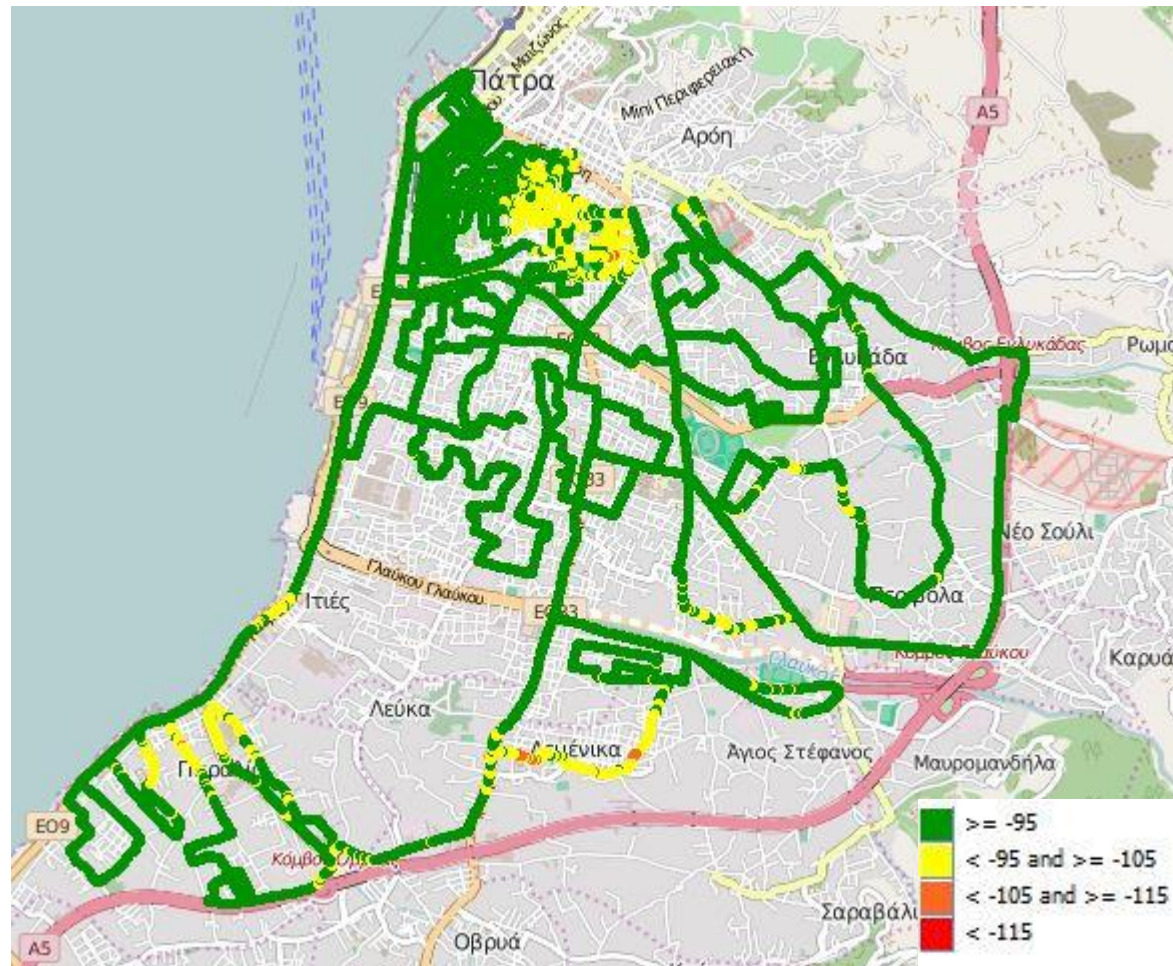
Εικόνα 13-2: Ραδιοκάλυψη WIND – UMTS
