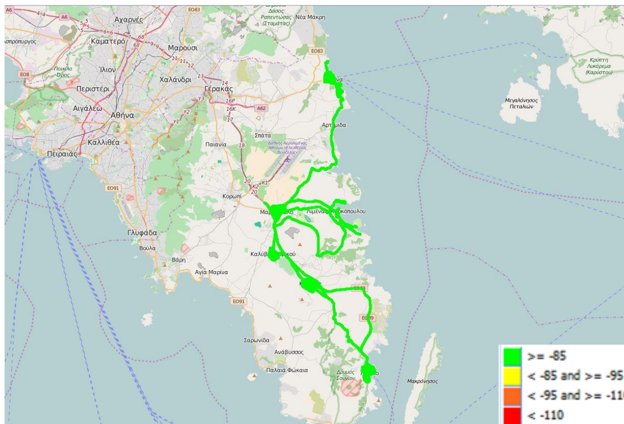
Εικόνα 13-1: Ραδιοκάλυψη WIND – GSM
